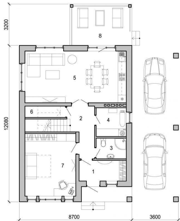
План первого этажа
