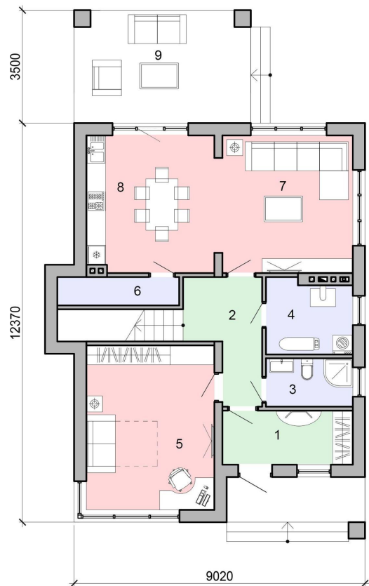
План первого этажа
