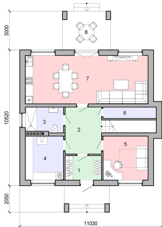
План первого этажа
