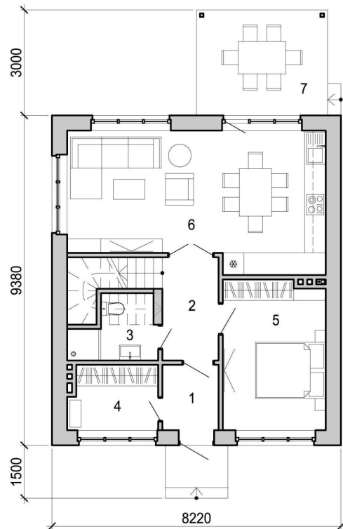
План первого этажа
