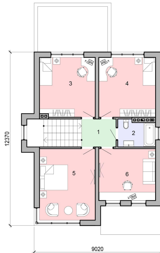
План второго этажа
