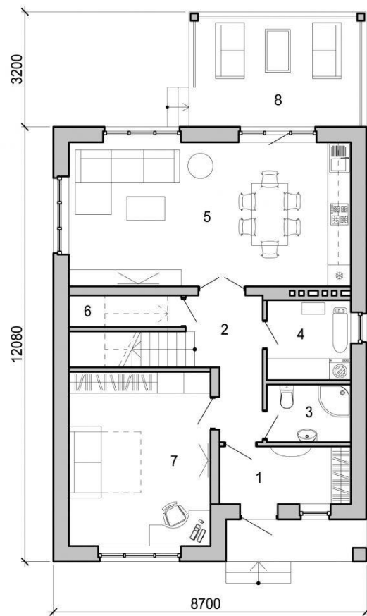
План первого этажа
