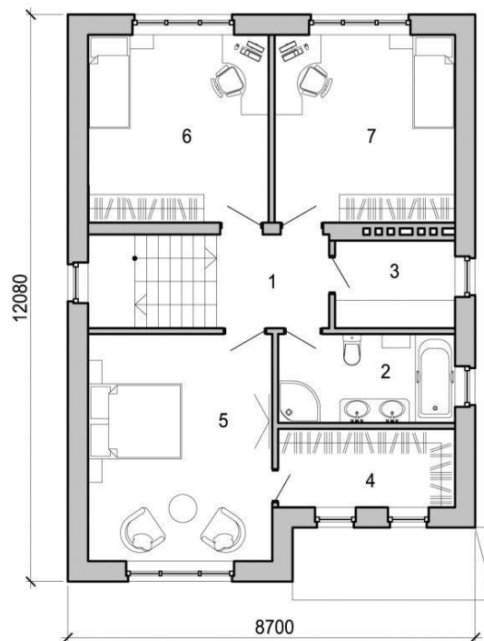
План второго этажа
